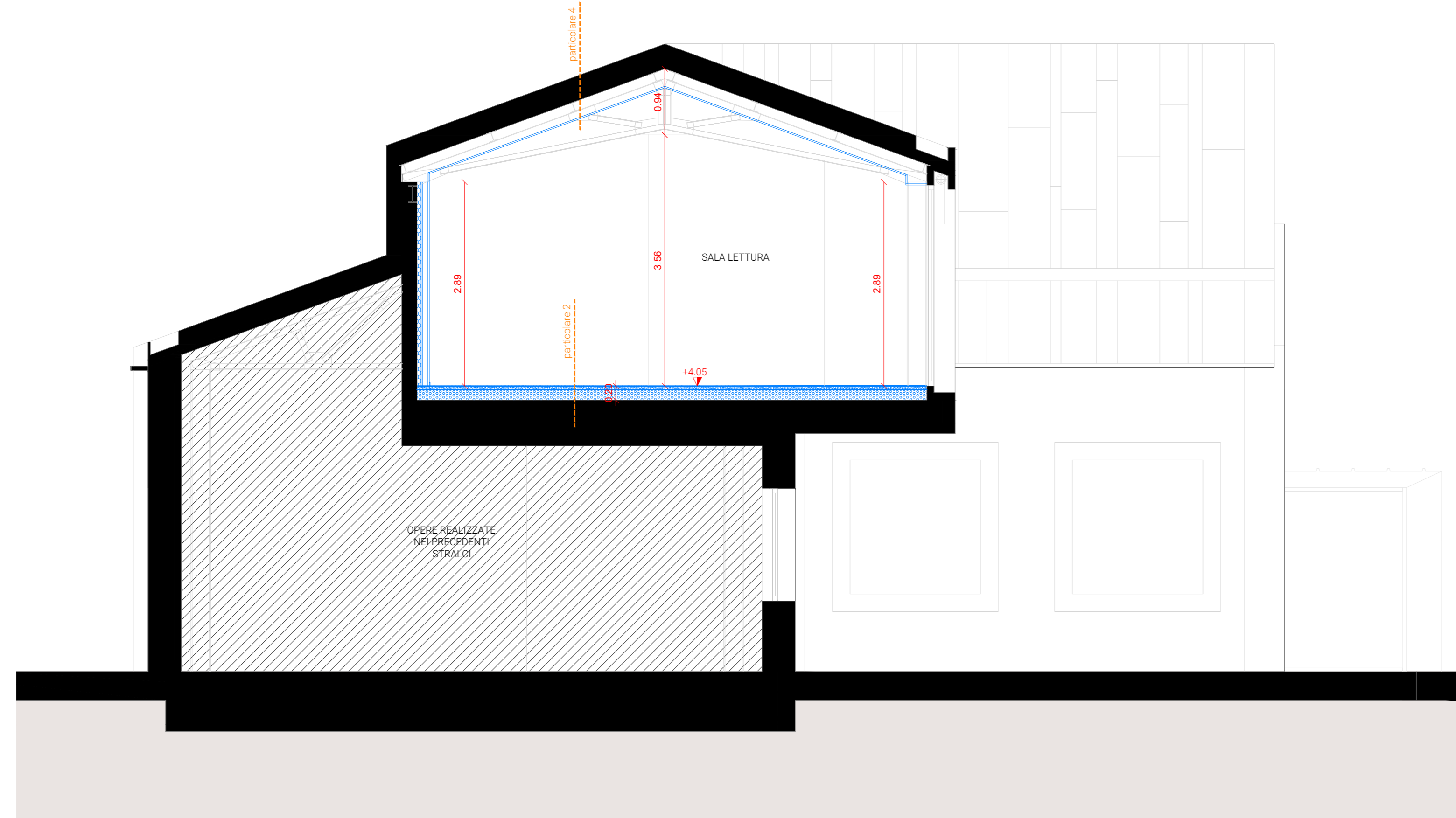
sezione C-C scala 1:50
