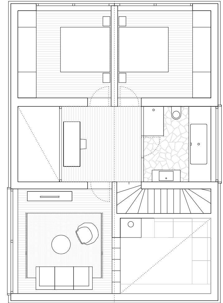
DACHGESCHOSS
