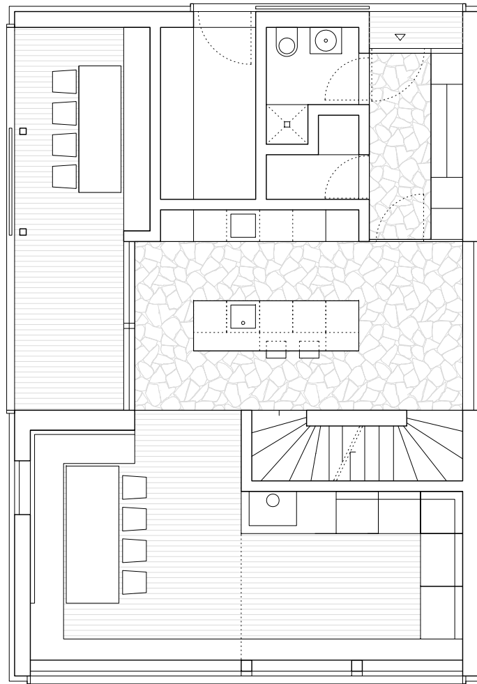
ERDGESCHOSS
