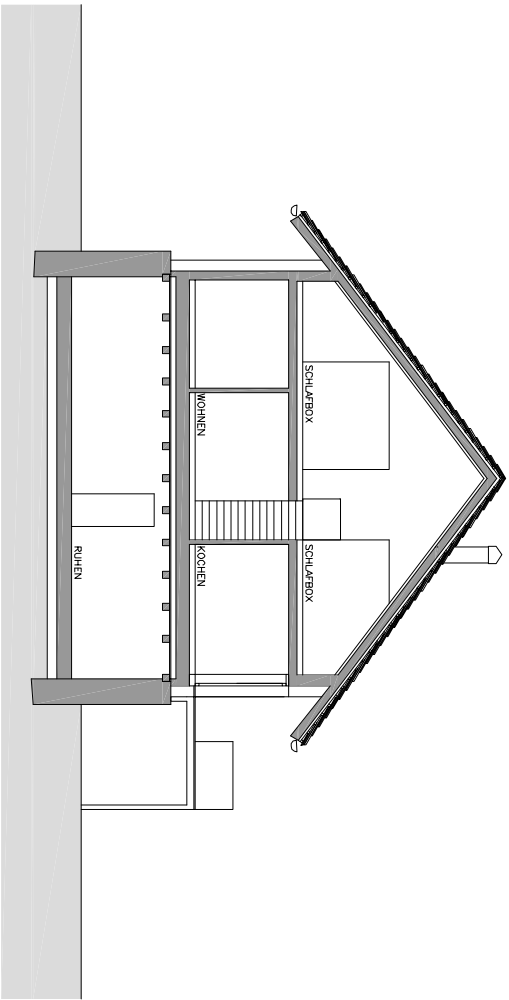
SCHNITT SEZIONE 0m 2m 4m 6m
