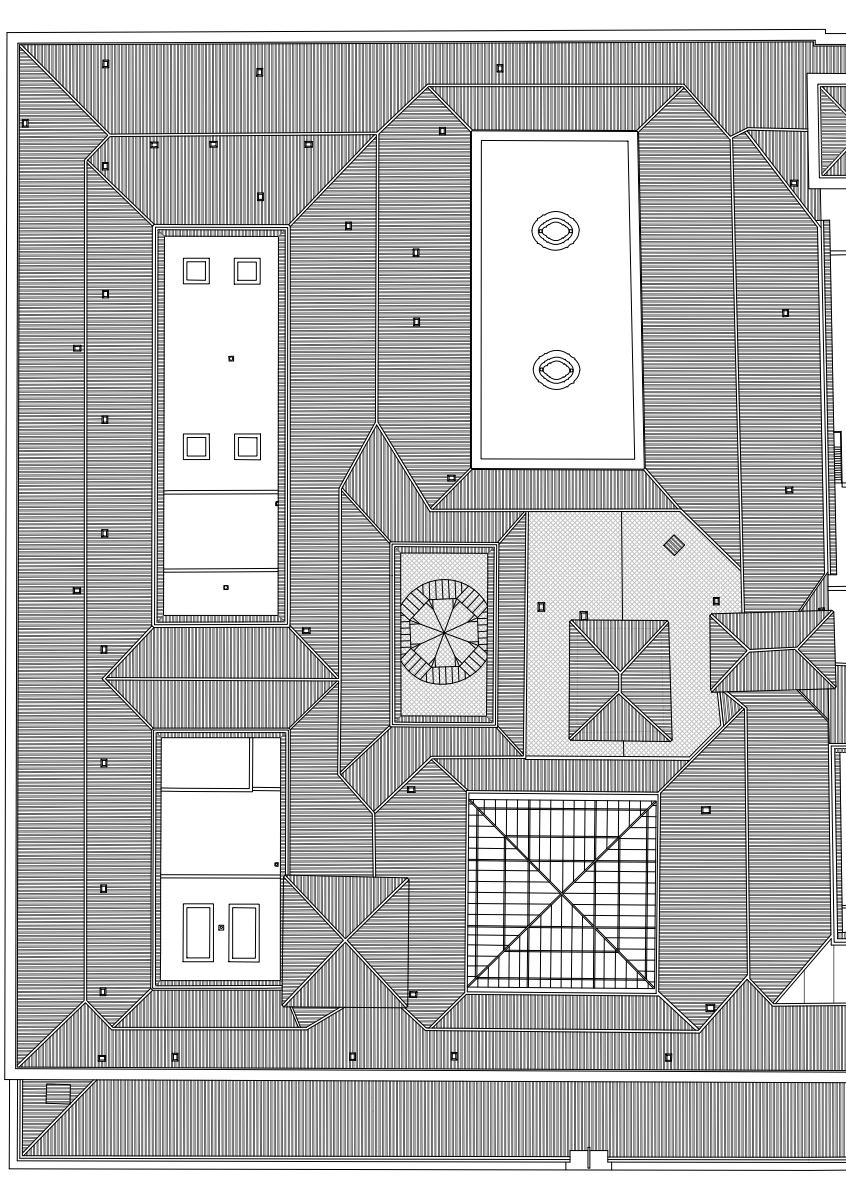
PLANTA CUBIERTA ESTADO PREVIO
