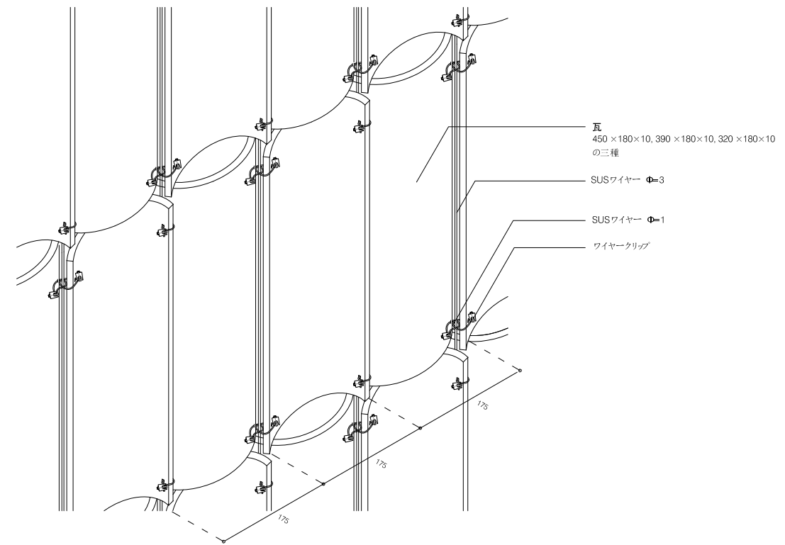
B1エントランス瓦スクリーン 裏面
