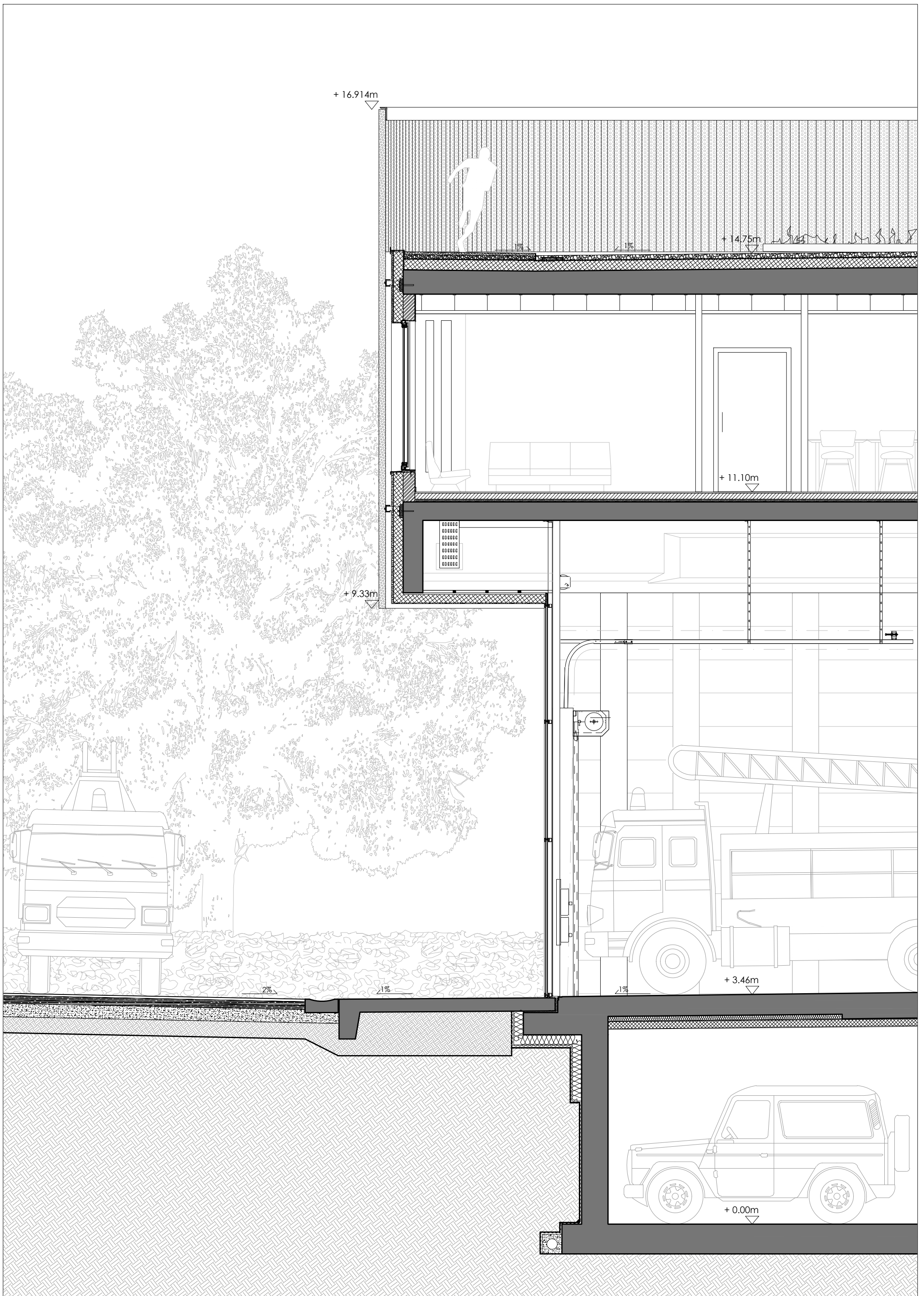
Coupe façade camions
