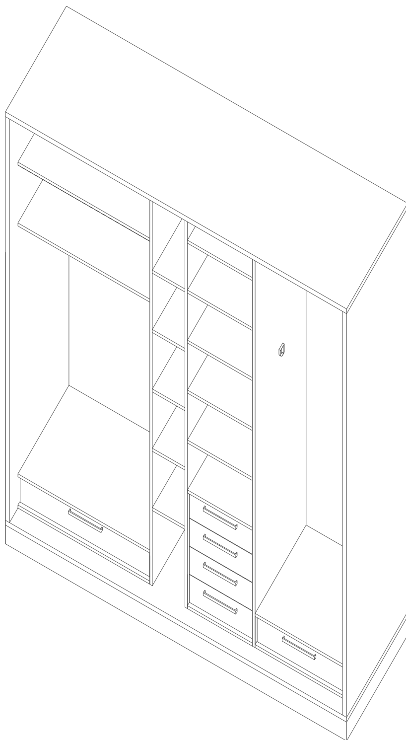
АКСОНОМЕТРИЈА М= 1: 20
