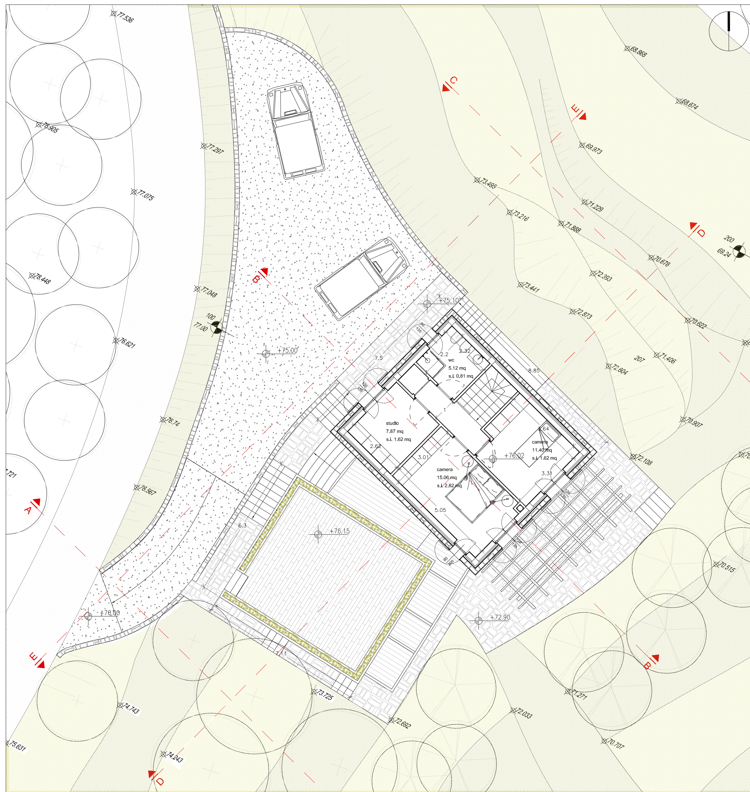
piano primo 1_100
