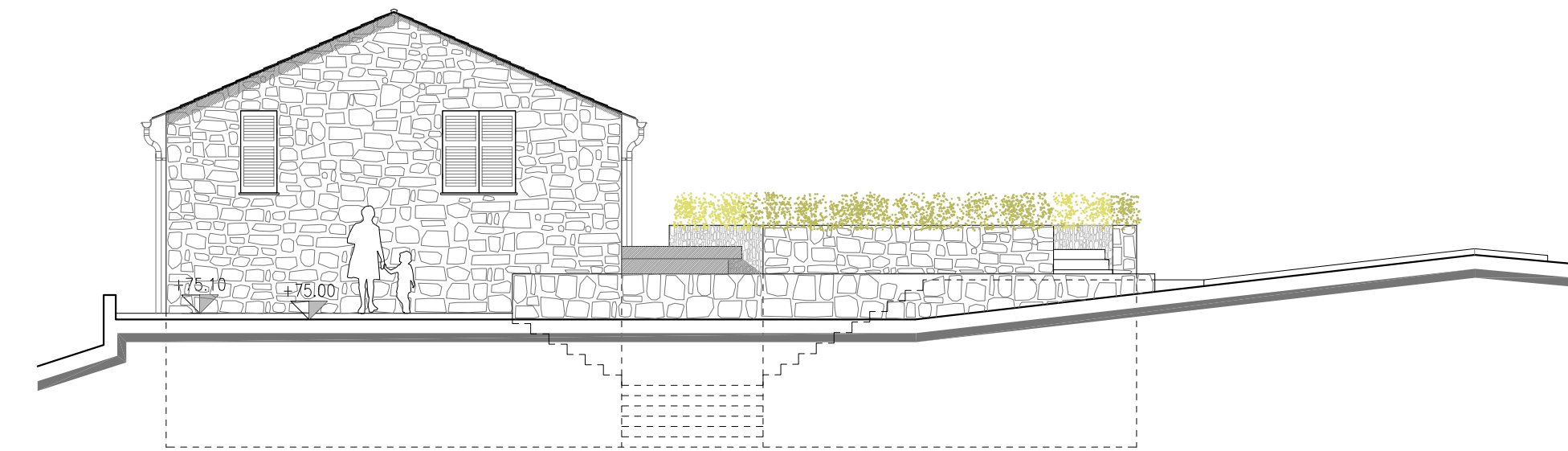
SEZ E-E_prospetto nord-est 1_100
