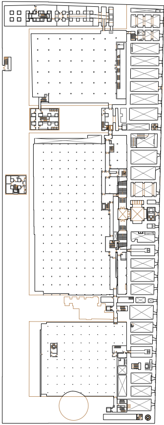
PLANTA SÓTANO -1
