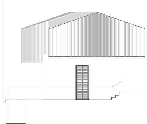
PROSPETTO EST
