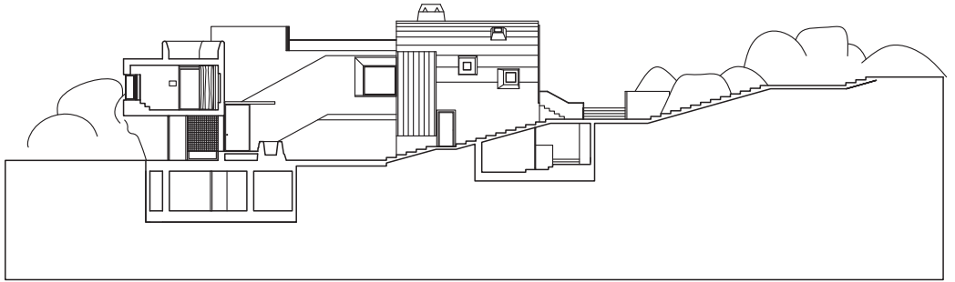
COUPE D-D
