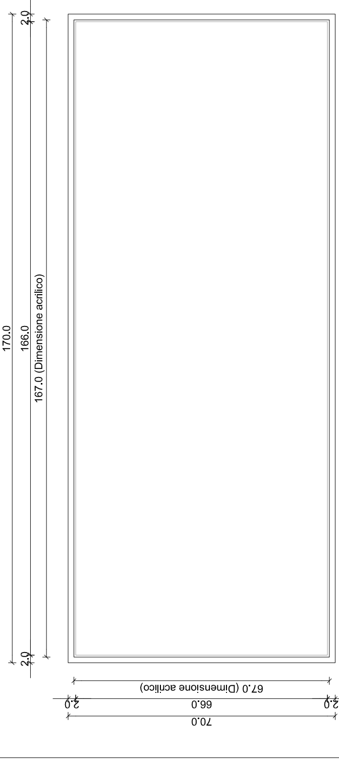
VISTA FRONTALE
