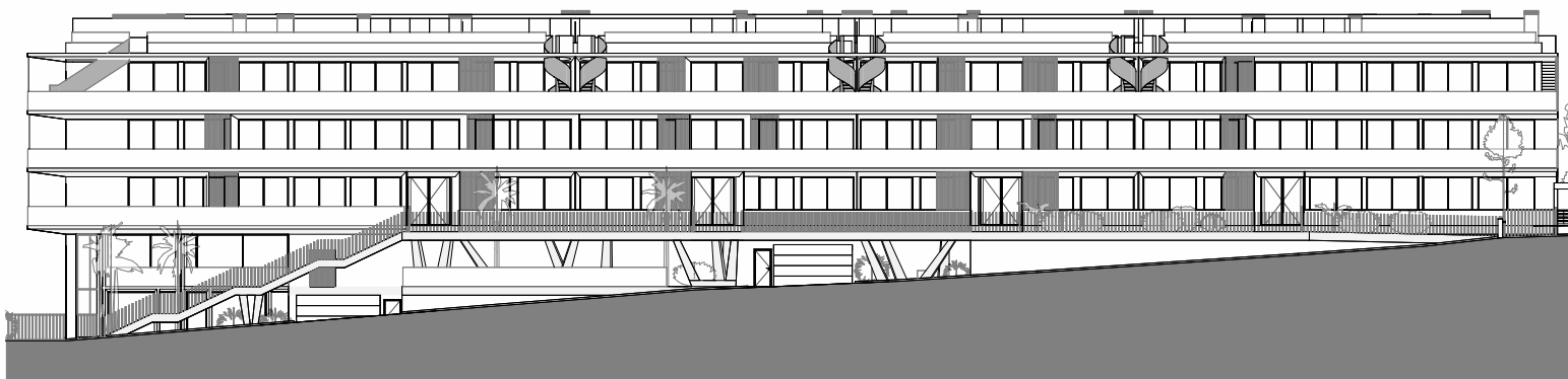
ALÇADO SUL
