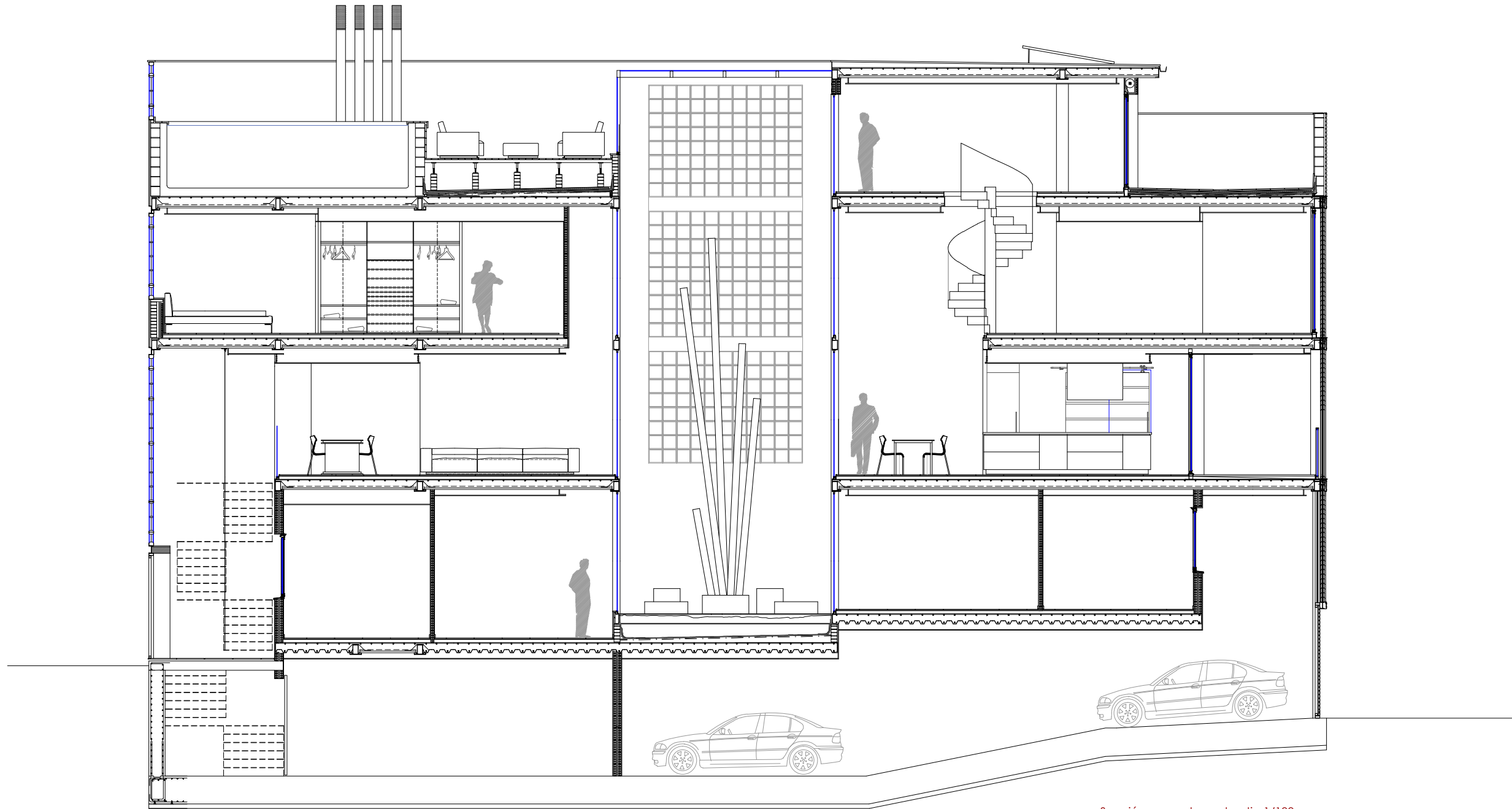
Sección general por el patio 1/100
