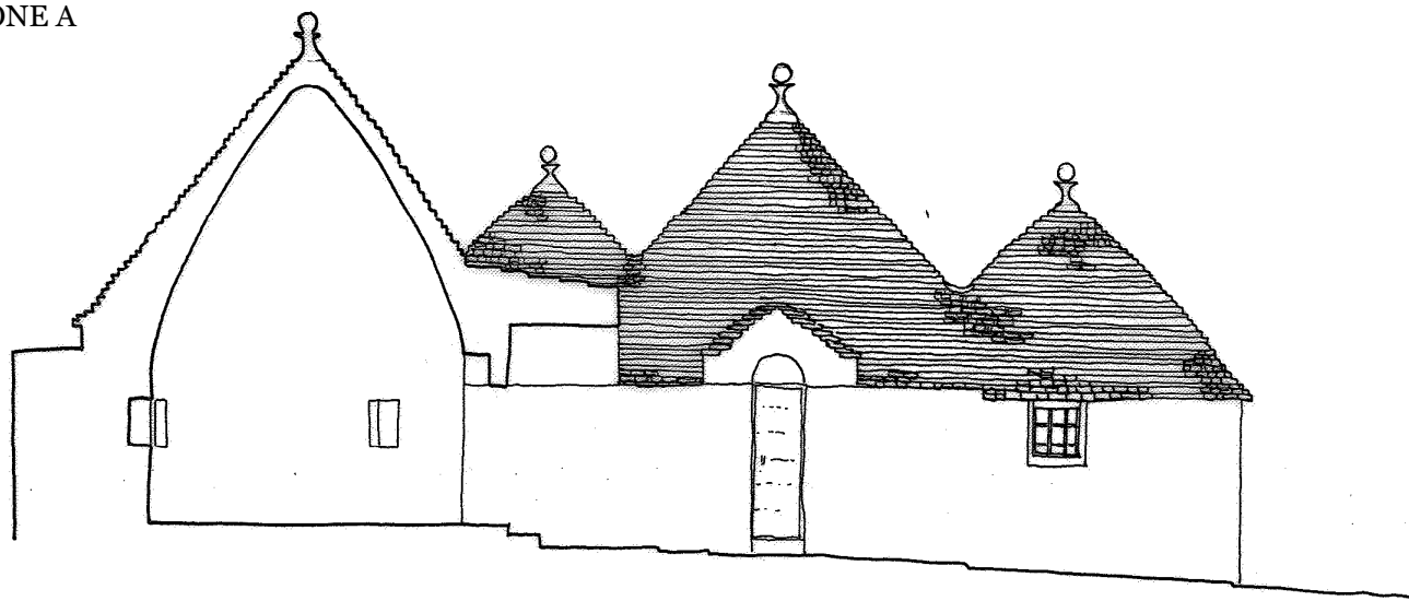
SEZIONE B
