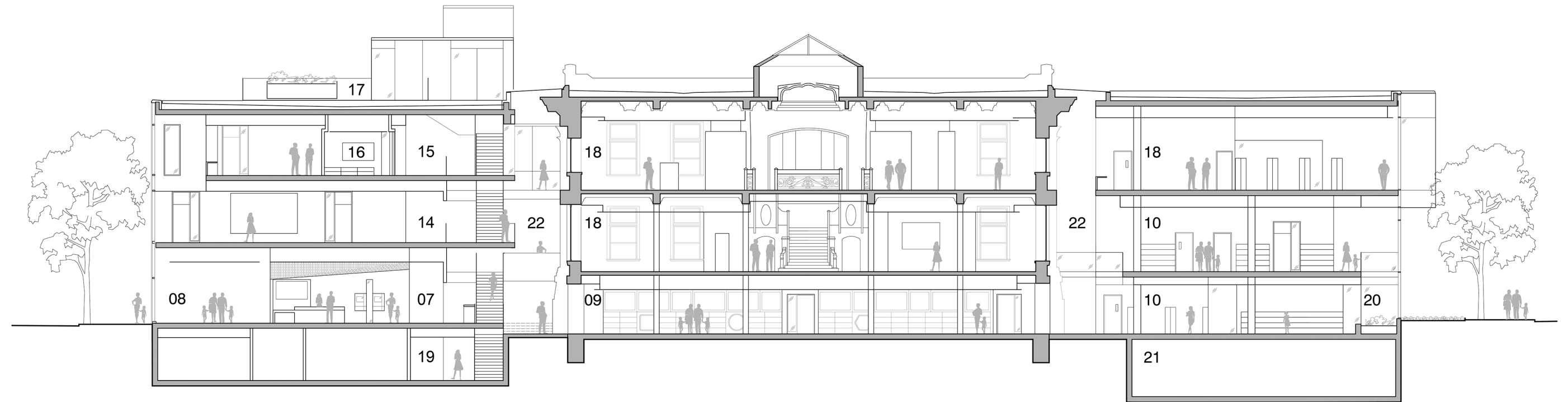
Coupe Longitudinale
