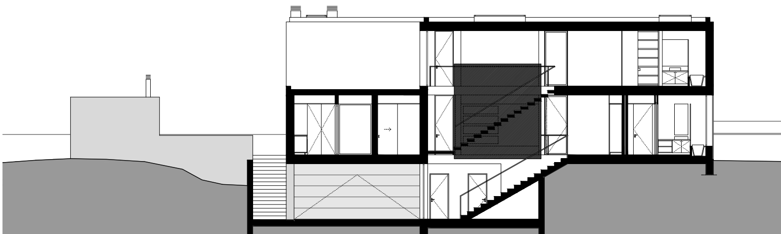
CORTE 1
