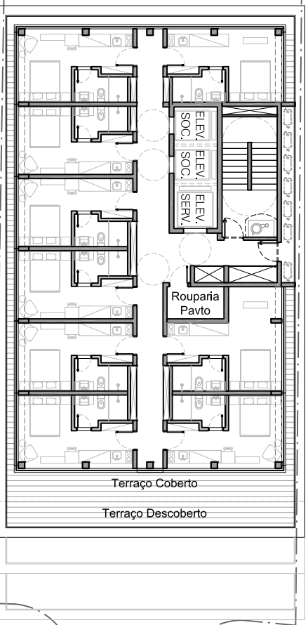
Planta 4º Pavimento ESC. 1/250
