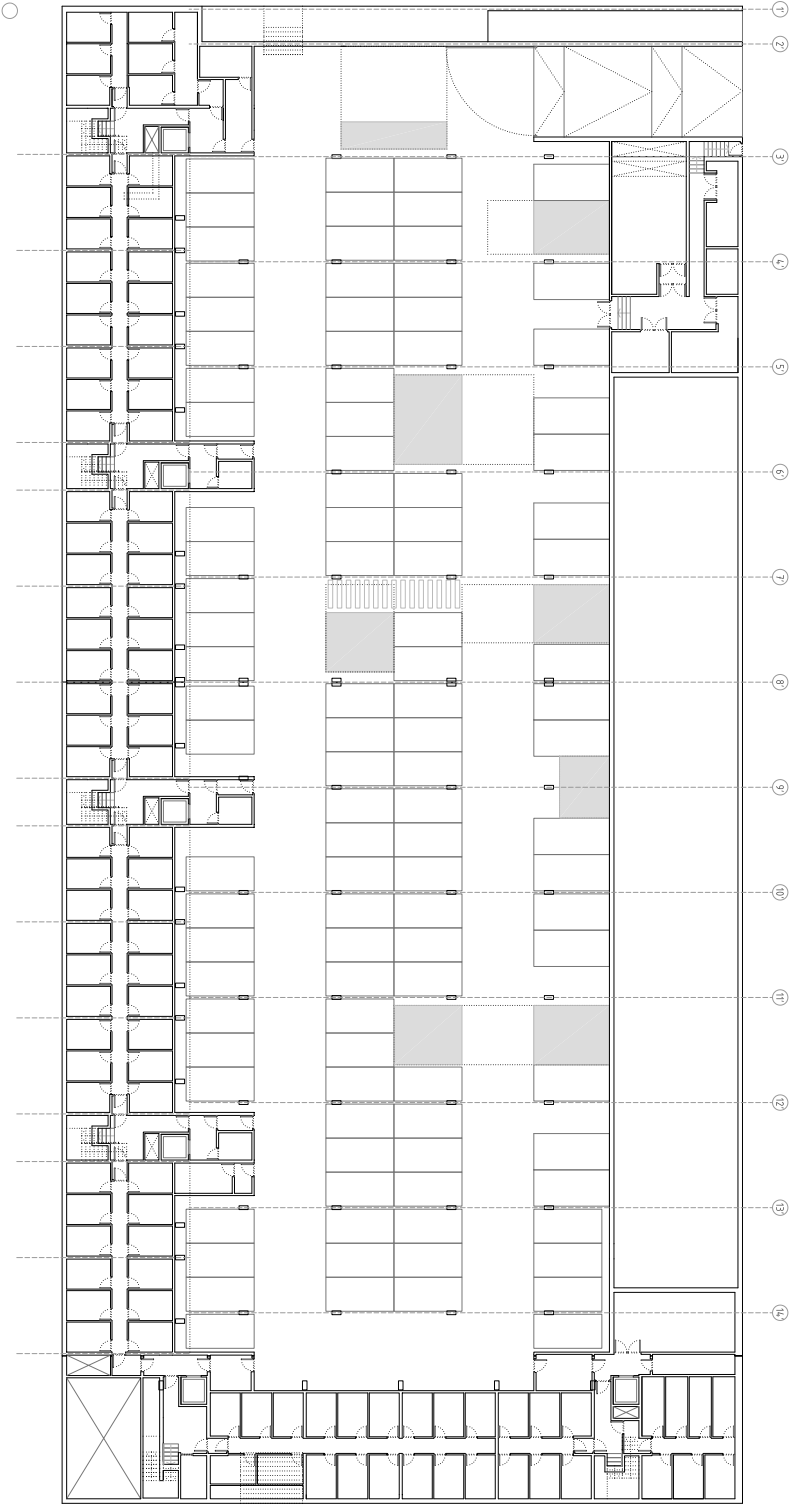
Planta Sótano 0 5 m
