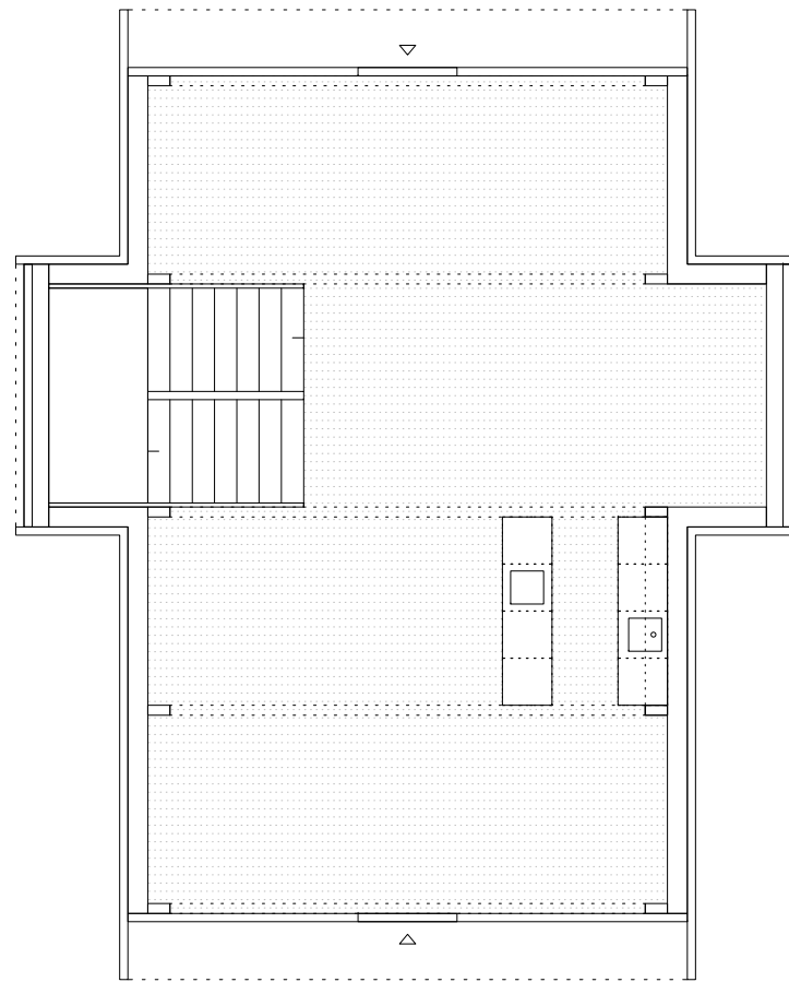
ERDGESCHOSS
