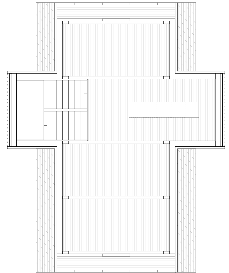
DACHGESCHOSS
