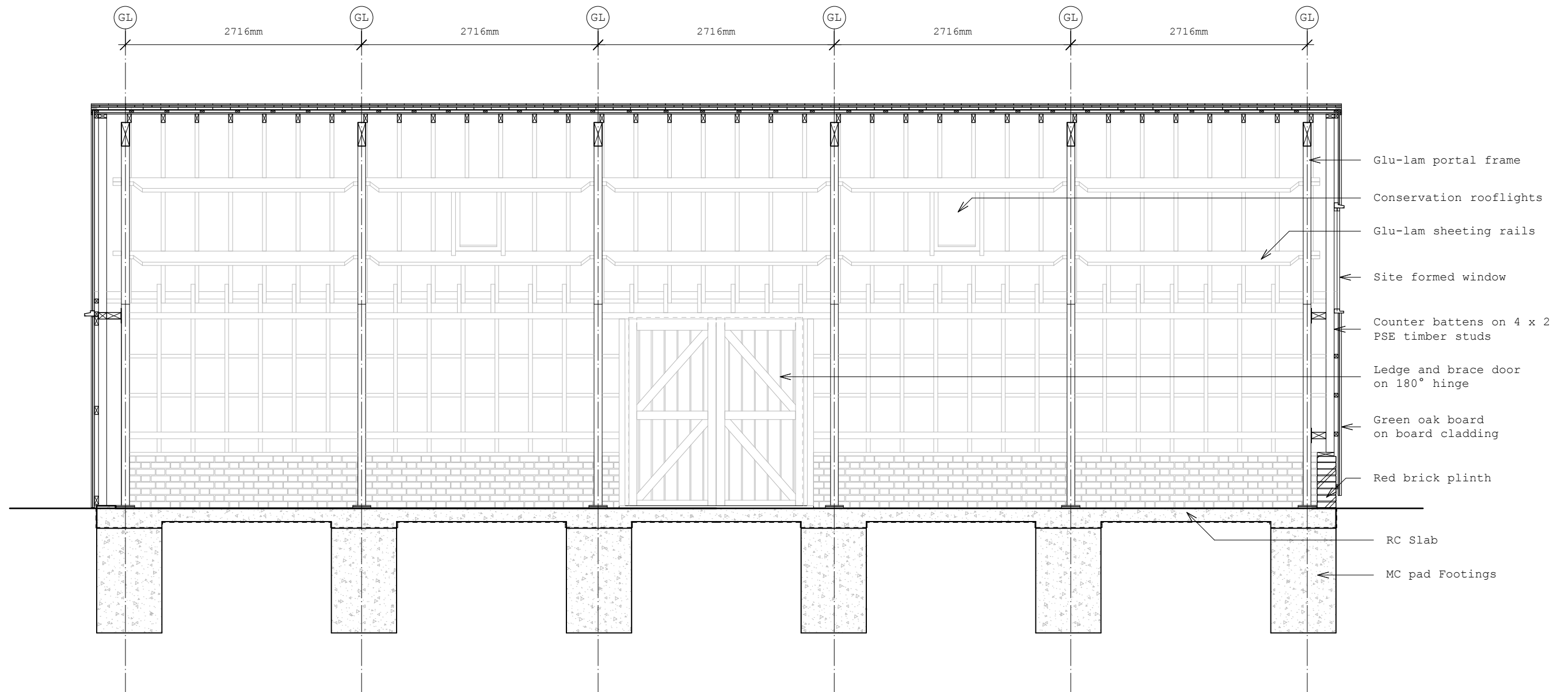
LONG SECTION 1:50 @ A3
