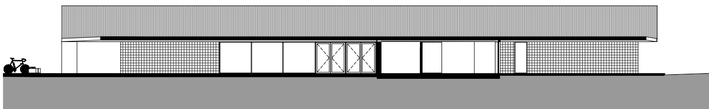
CORTE 11
