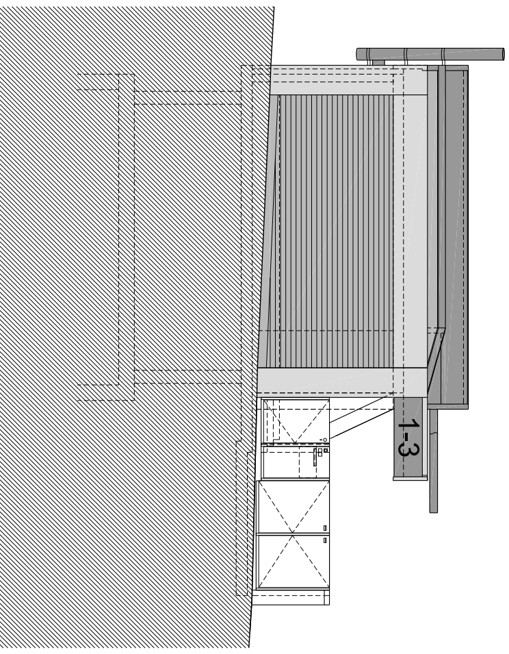
ansicht süd (garage)
