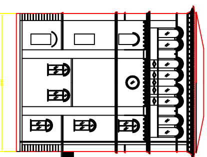
PROSPETTO NORD
