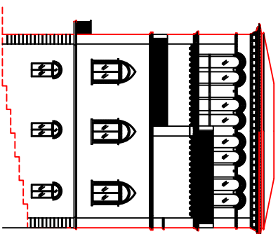
PROSPETTO SUD
