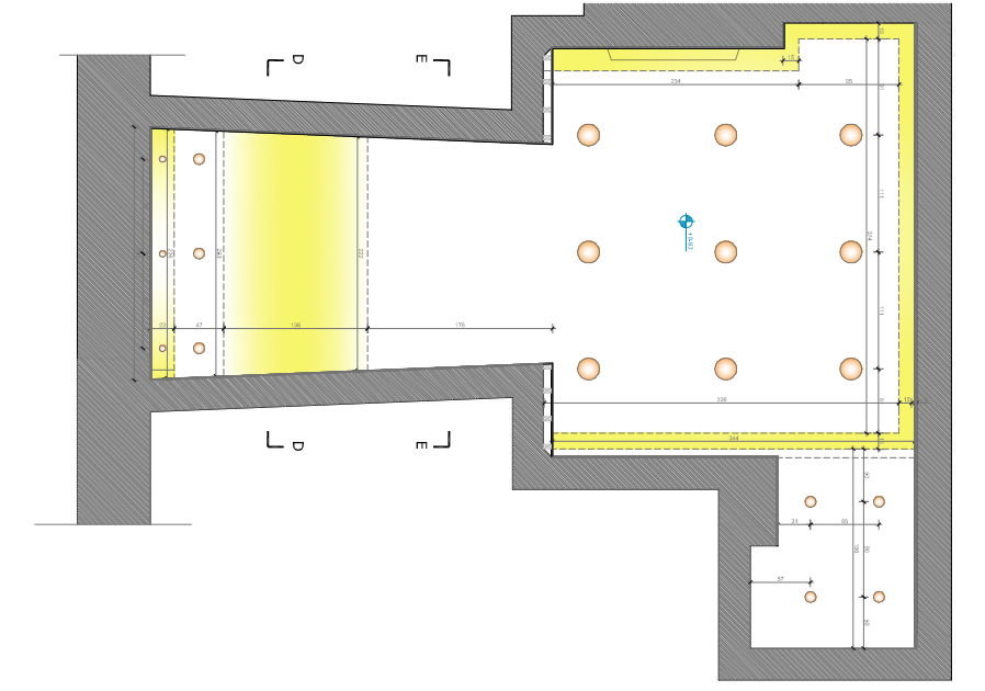
Planus componendi - scala 1:50
