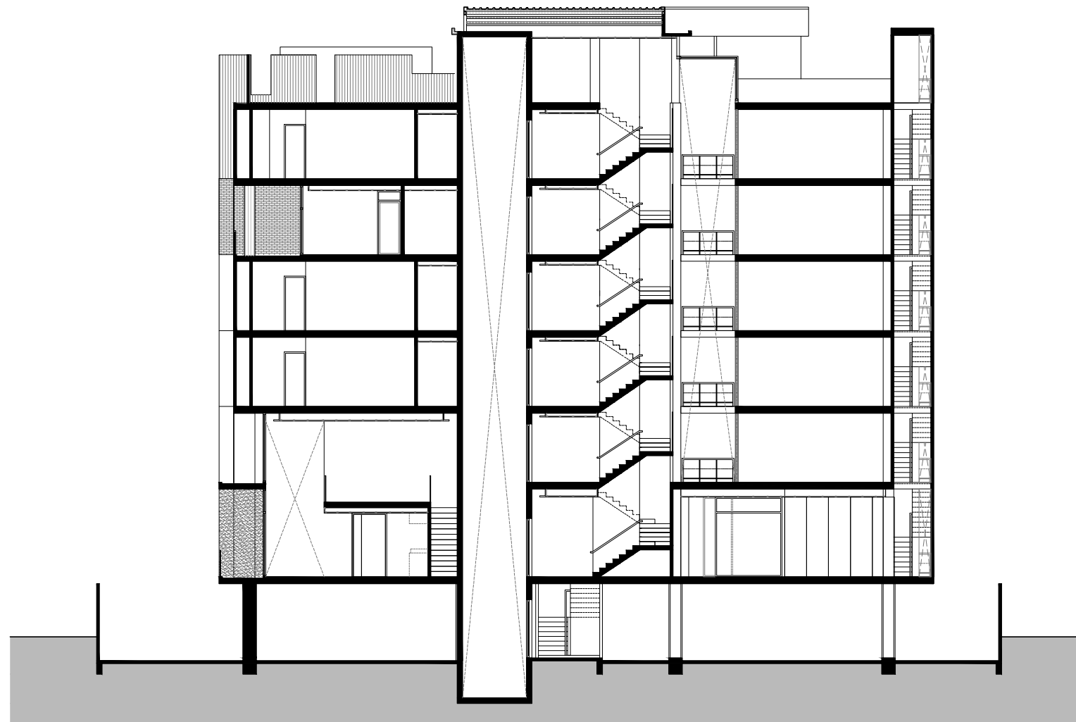
A-A SECTION
