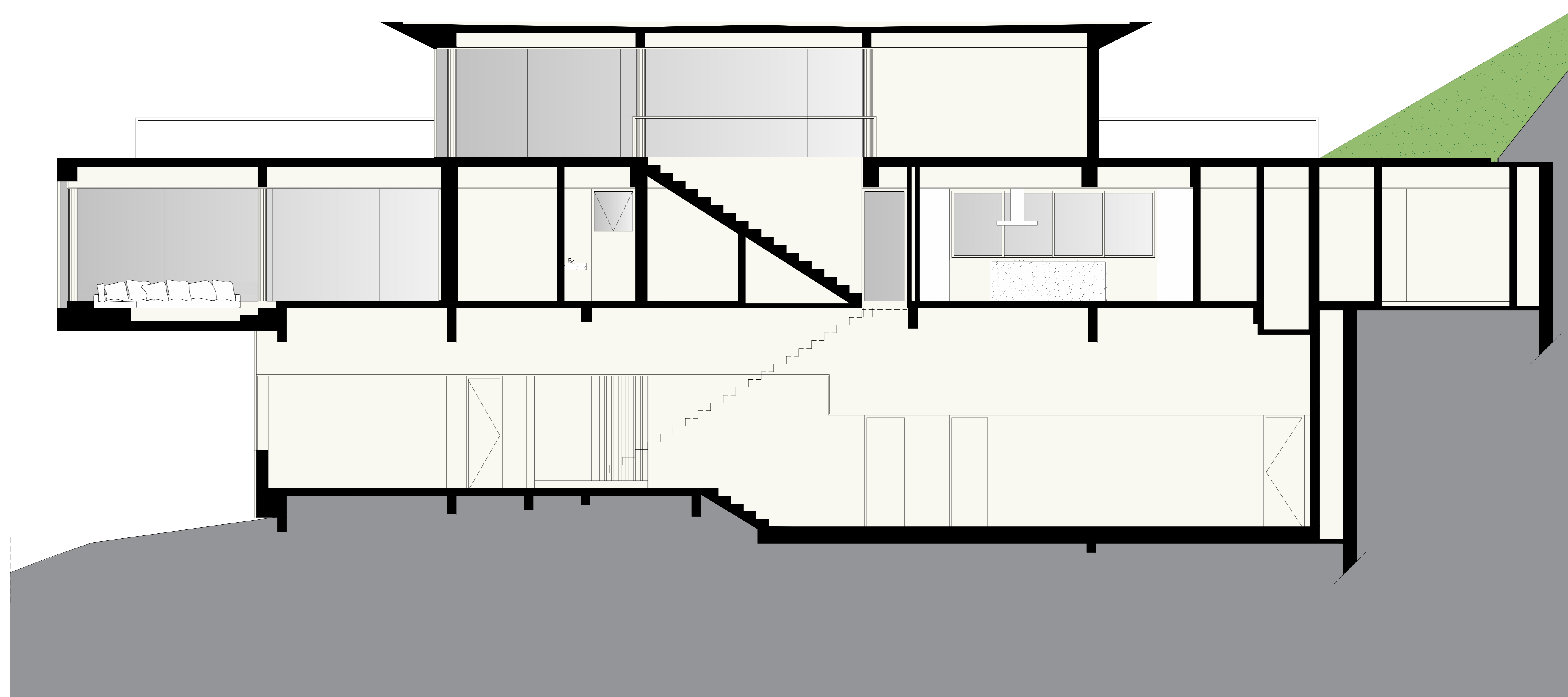
CORTE B
