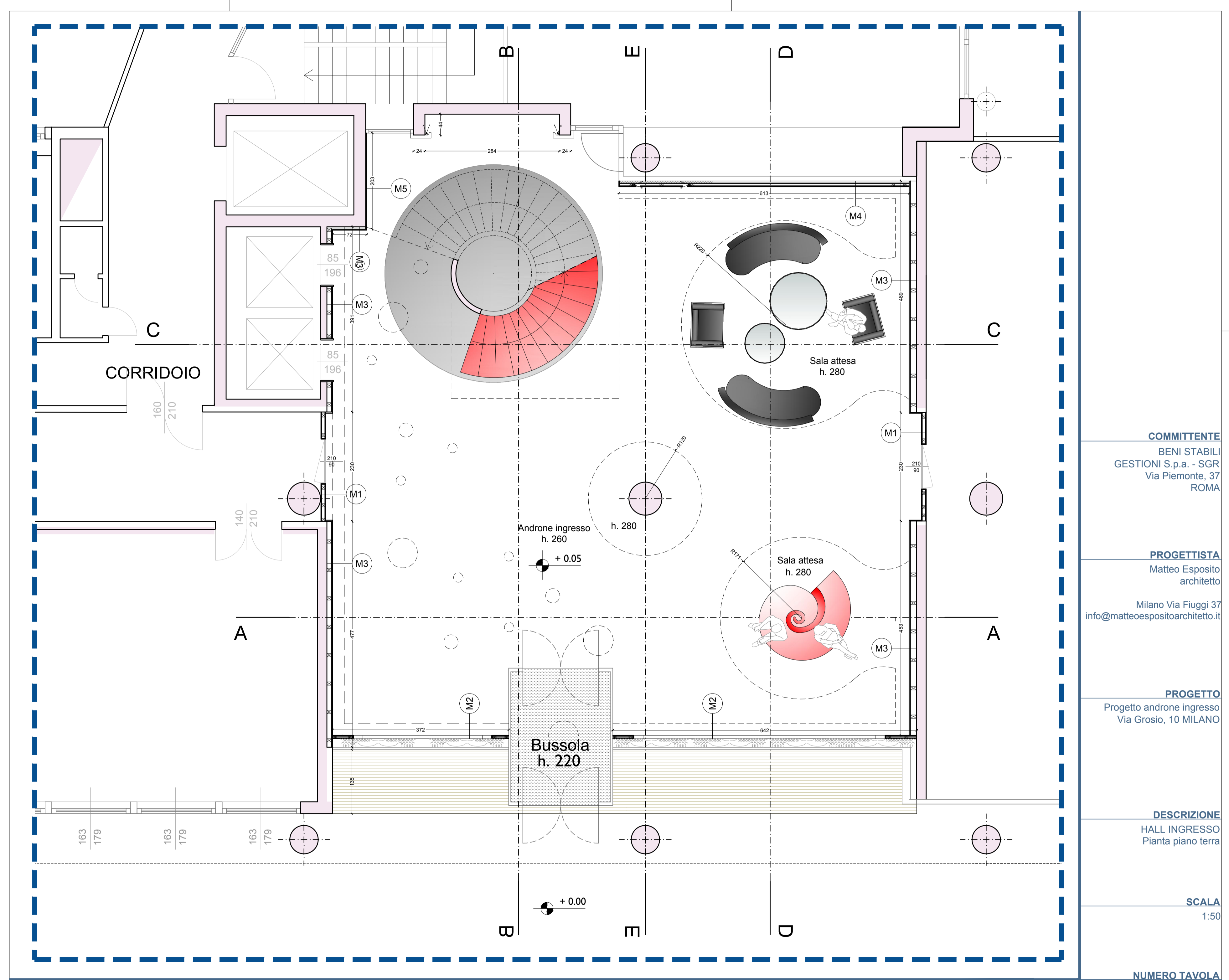
Pianta piano terra - scala 1:50
