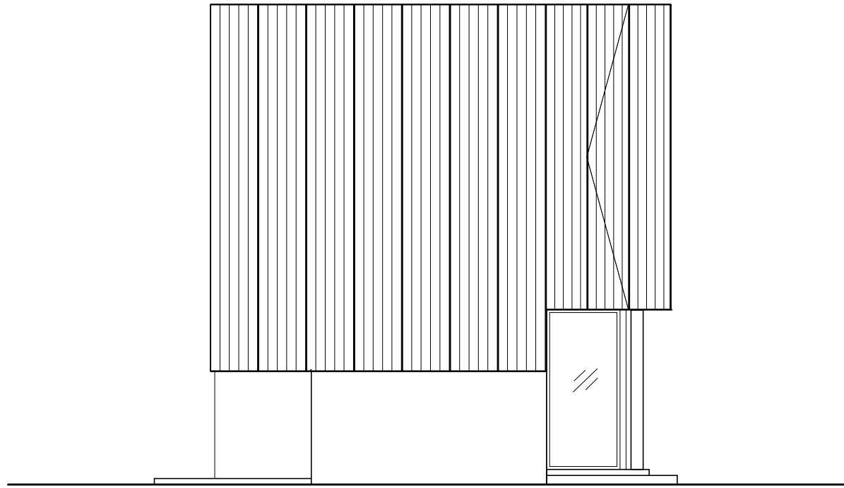
ELEVATION 1
