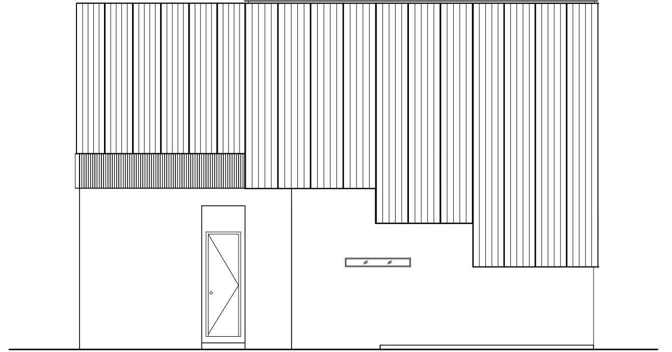
ELEVATION 2
