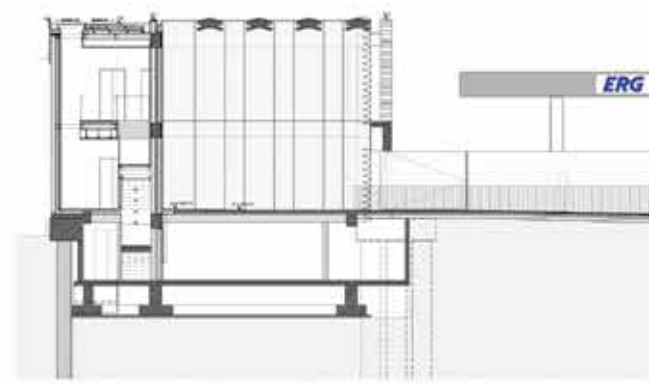
Sezione trasversale
