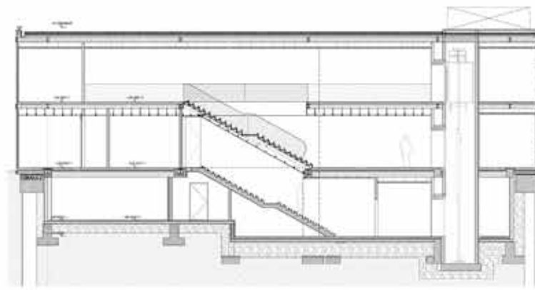
Sezione longitudinale
