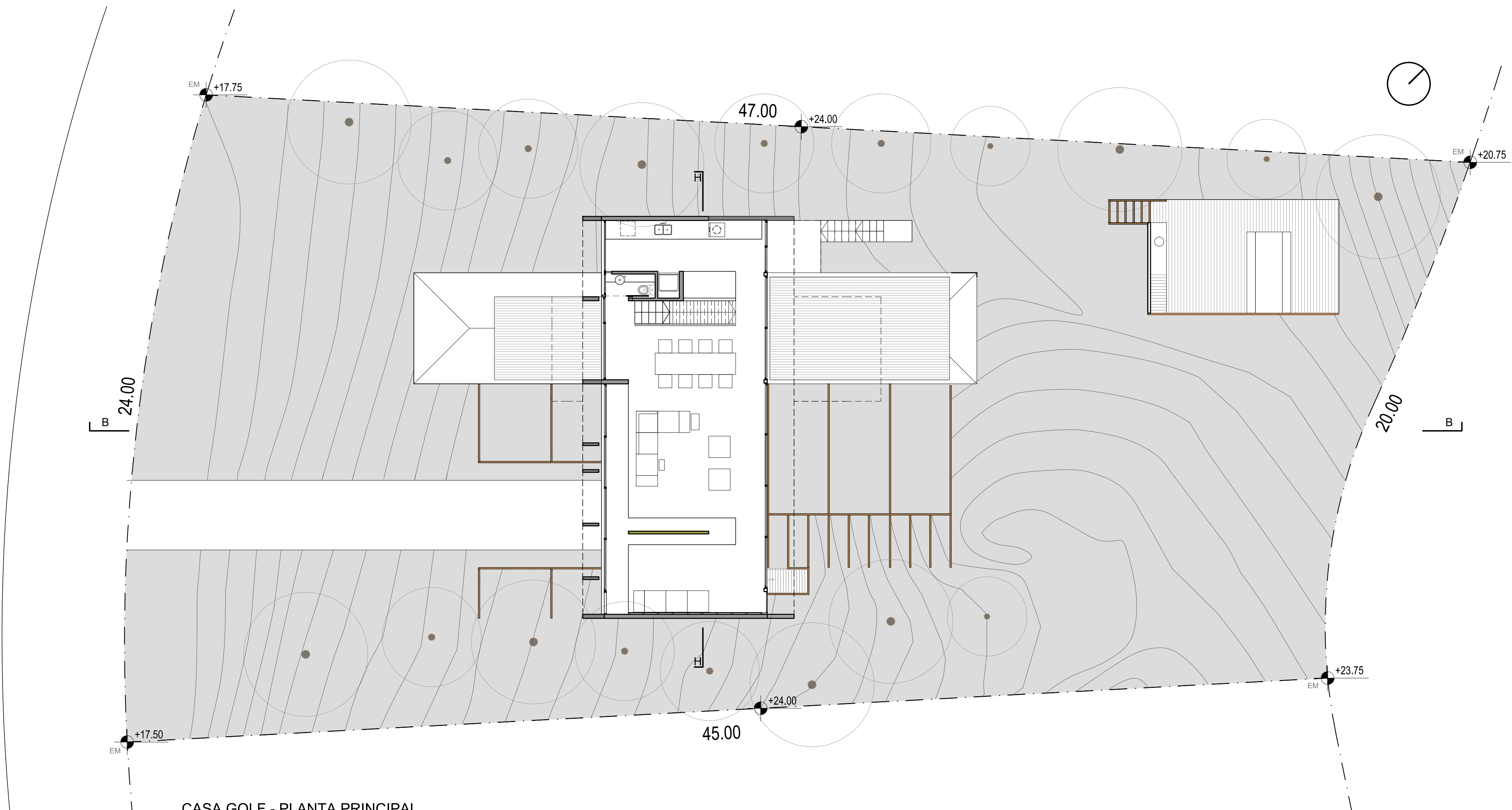
CASA GOLF - PLANTA PRINCIPAL
