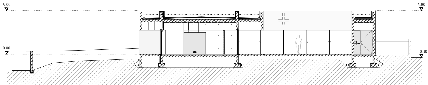
LONGITUDINAL SECTION 04
