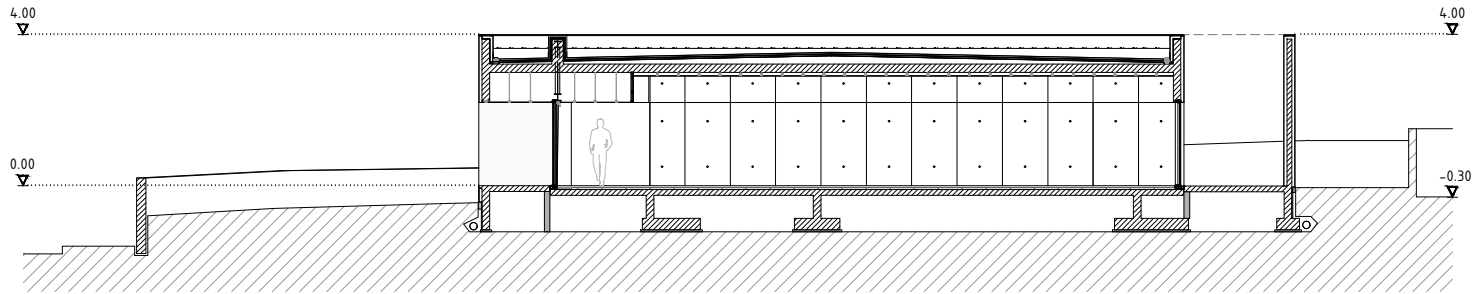
LONGITUDINAL SECTION 01
