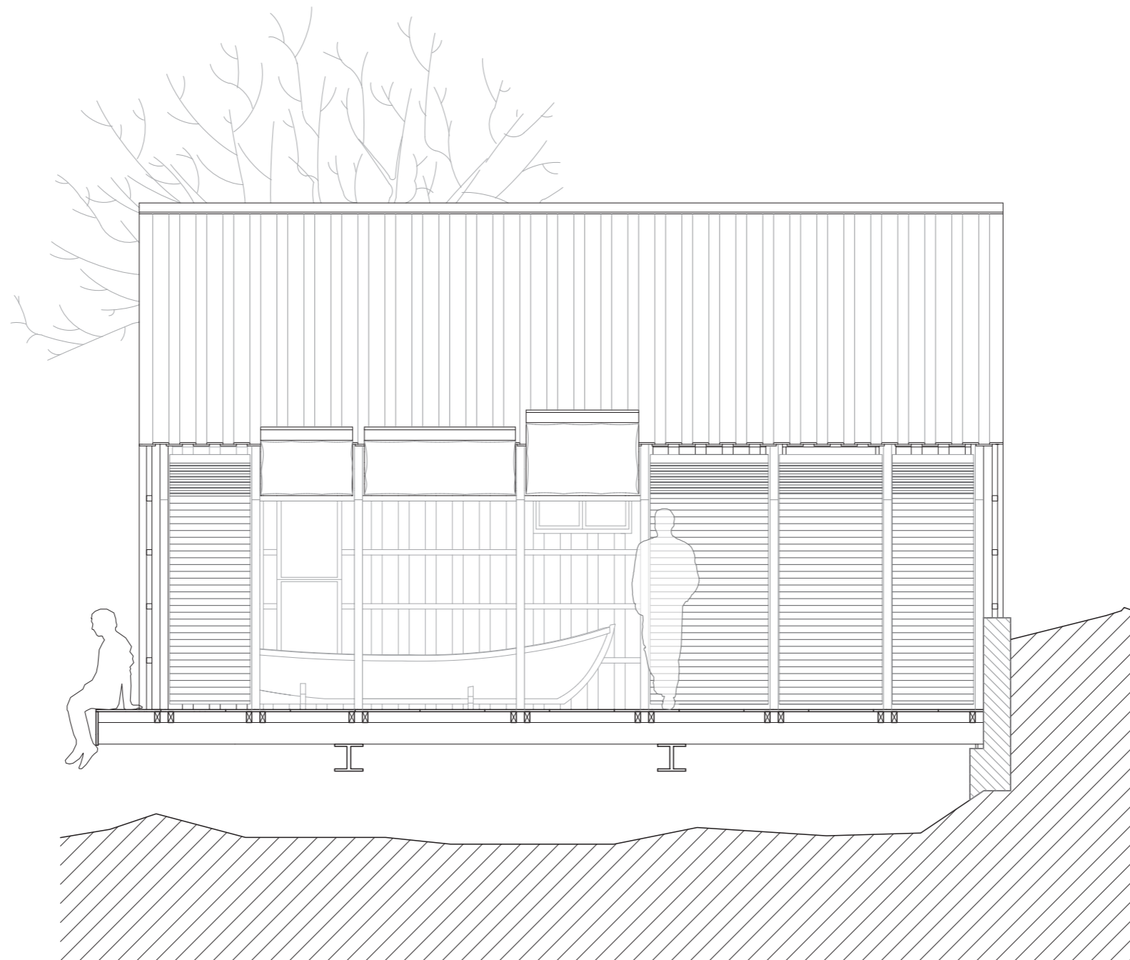
Fasade mot uteplass Målestokk 1:50
