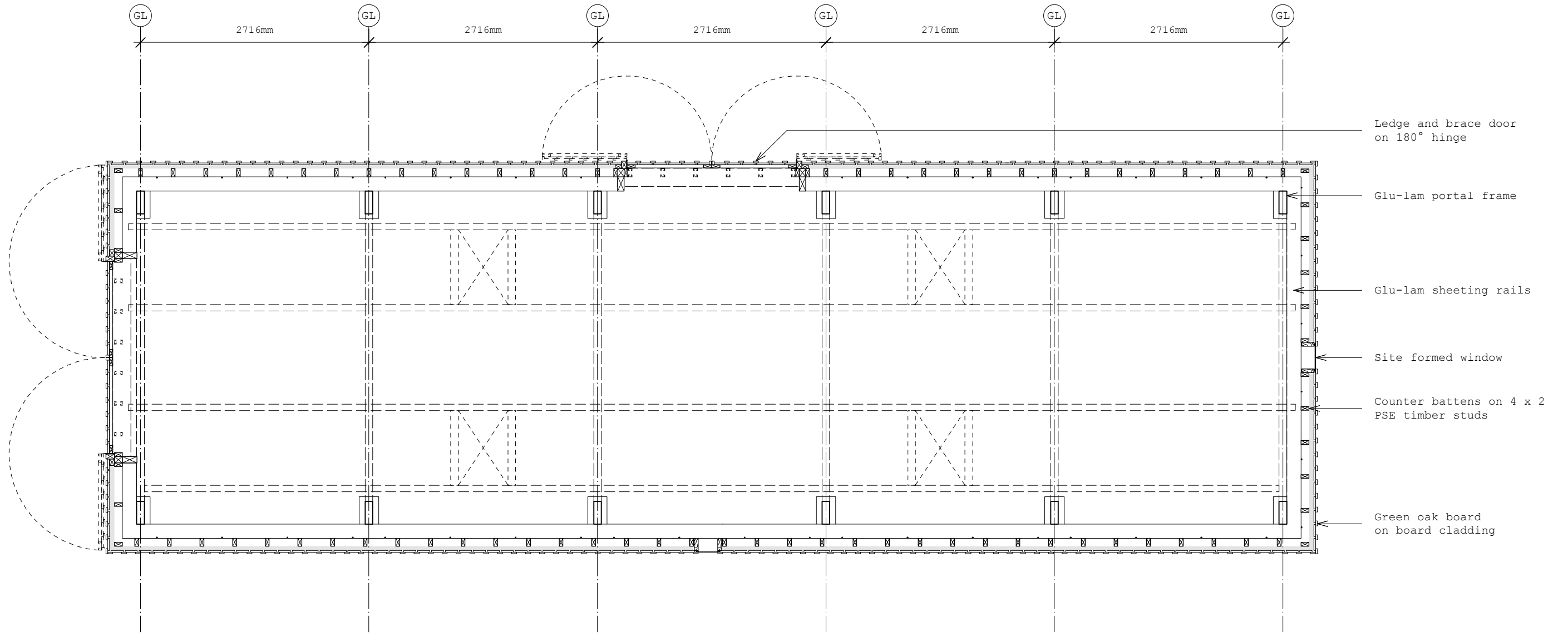
PLAN 1:50 @ A3
