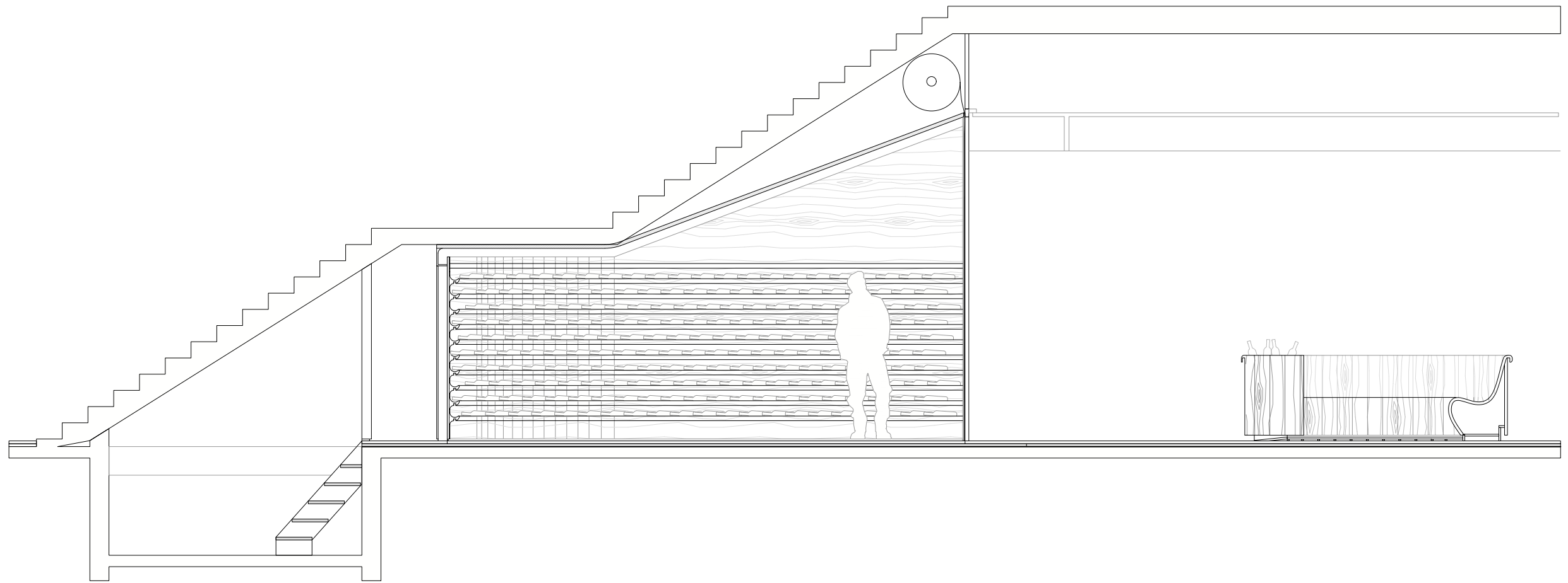
SECTION A-A
