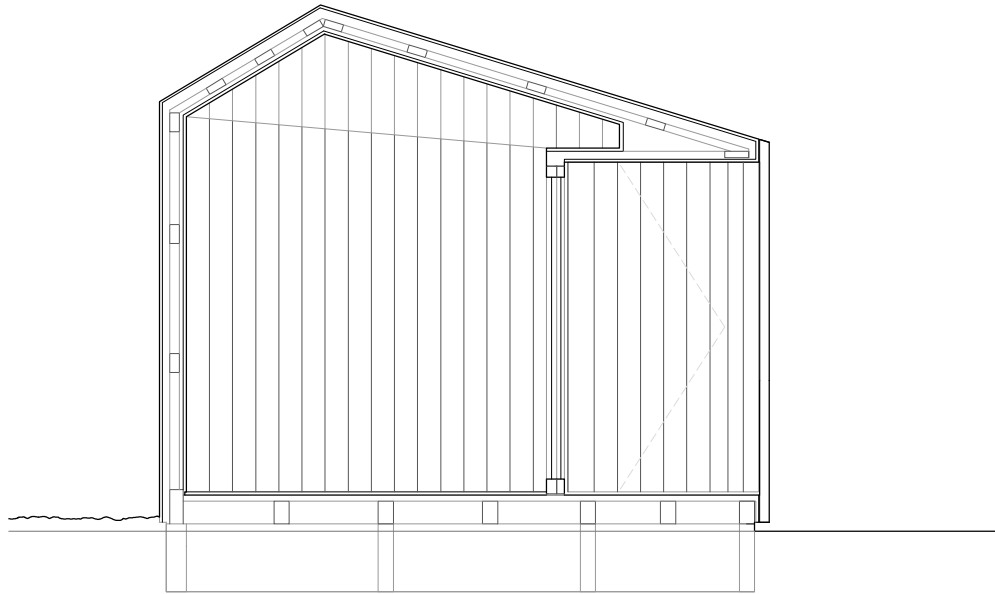
CORTE B
