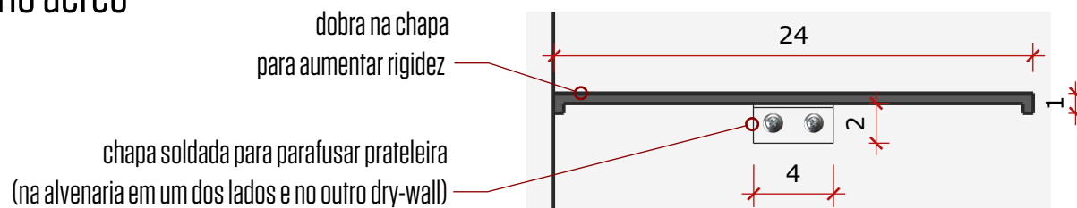
corte prateleira
