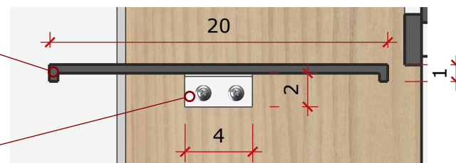
corte prateleira
