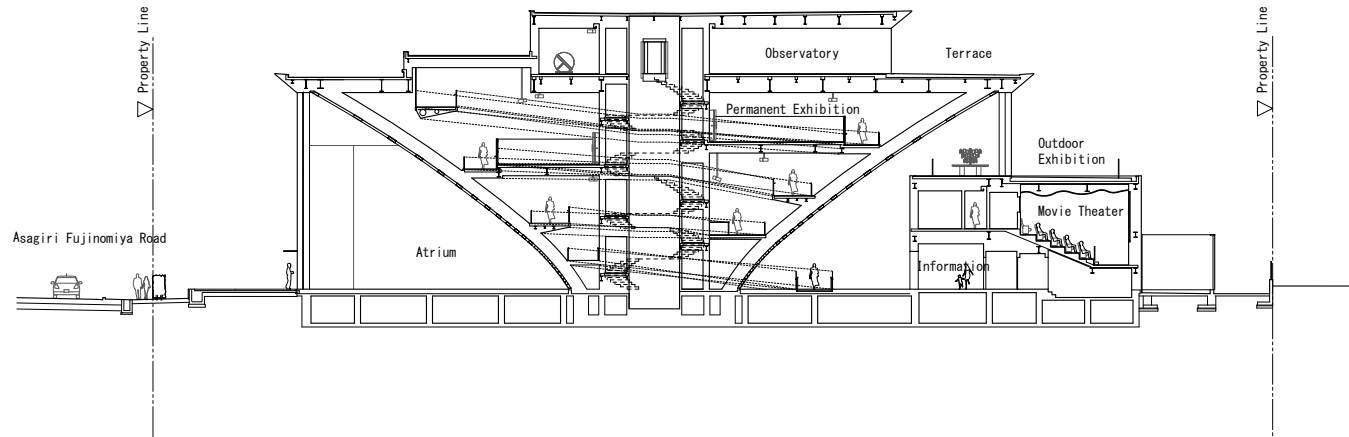
A-A' Long Section 1:500
