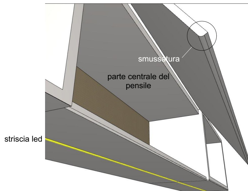
Dettaglio anta a vasistas
