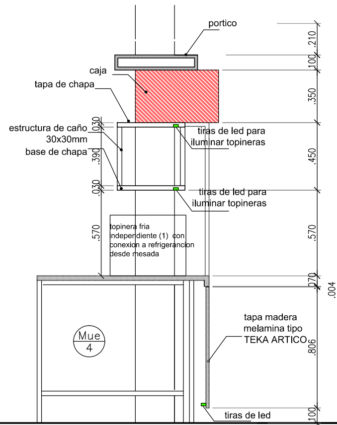
CORTE 1-1
