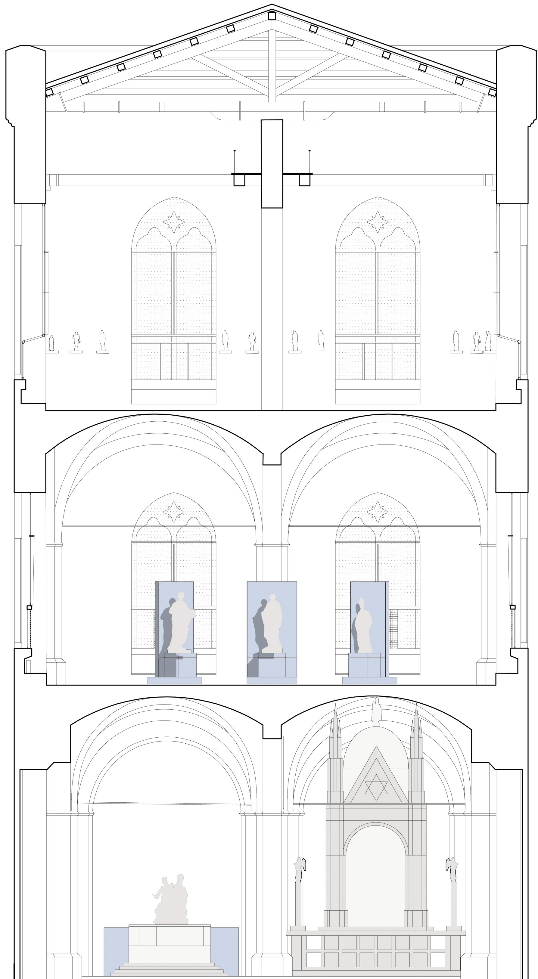
Sezione CC'
