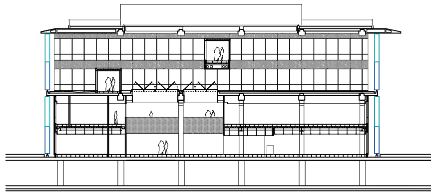
SECCIÓN 4
