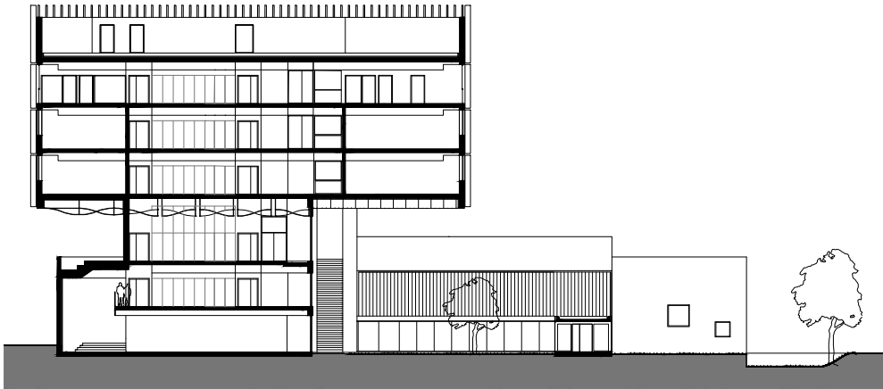
COUPE A-A
