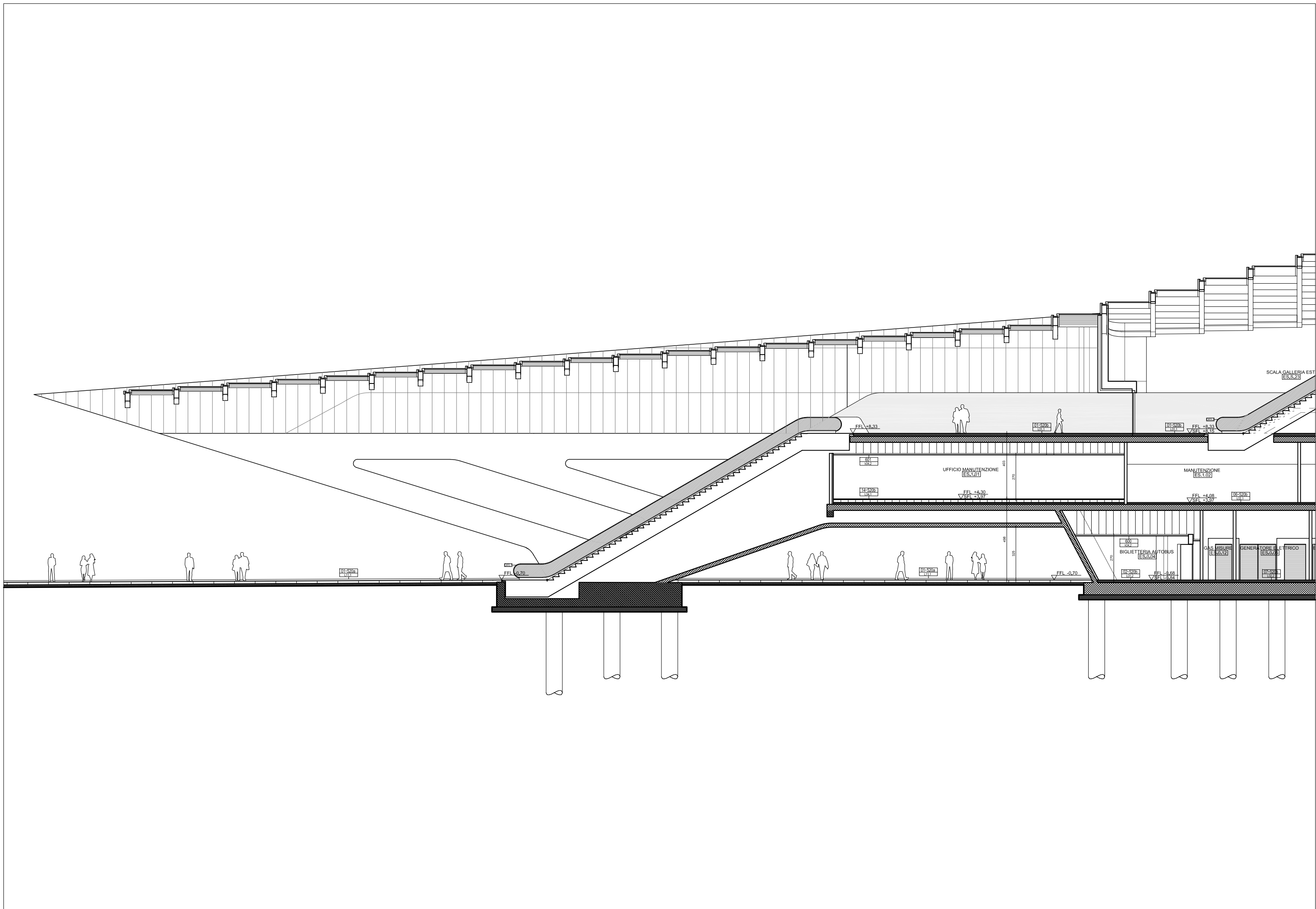
Sezione 231b
