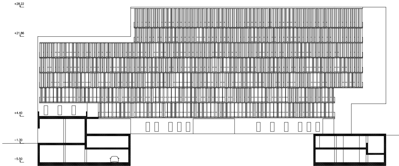
SECCIÓN D
