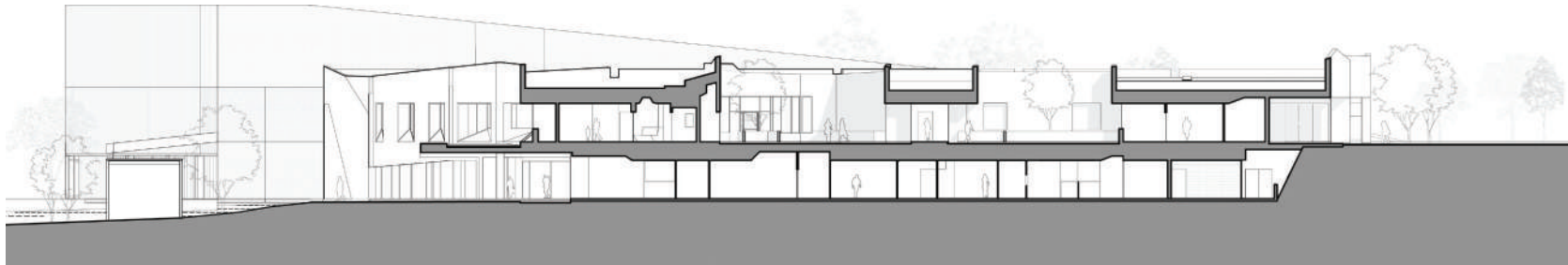
LONGITUDINAL SECTION 1:500
