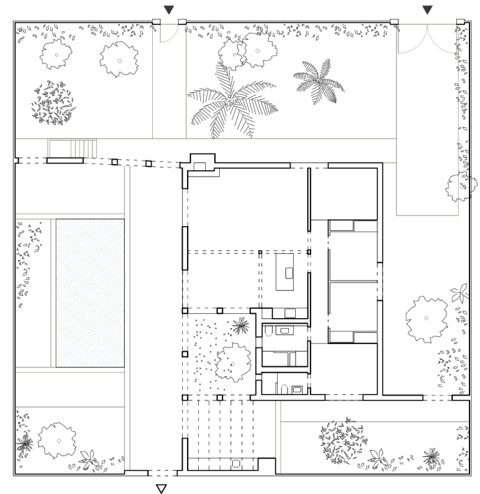
Propuesta 1/300
