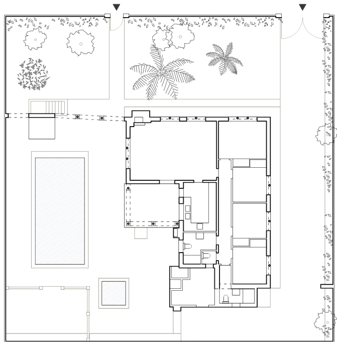
Estado original 1/300
