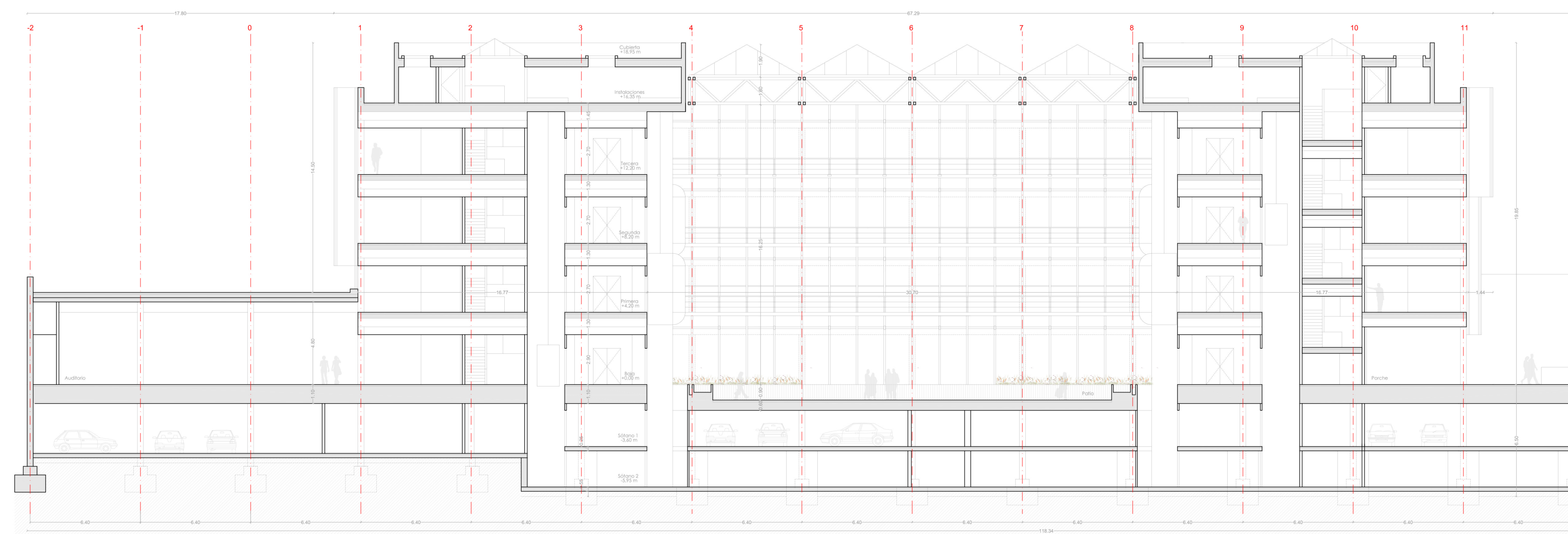
SECCIÓN BB
