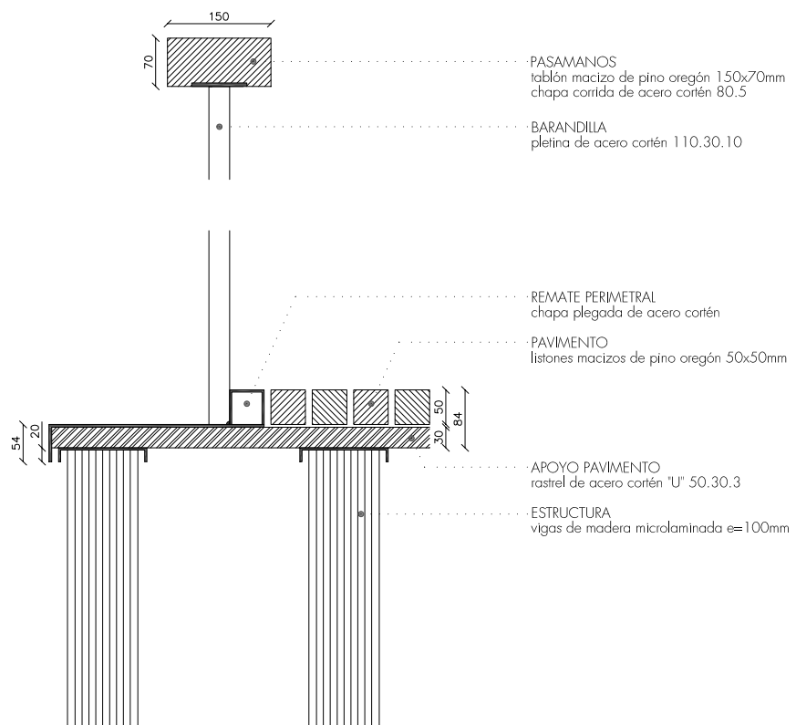
MIRADOR - VOLADIZO DE MADERA MICROLAMINADA SECCIÓN CONSTRUCTIVA POR BARANDILLA
