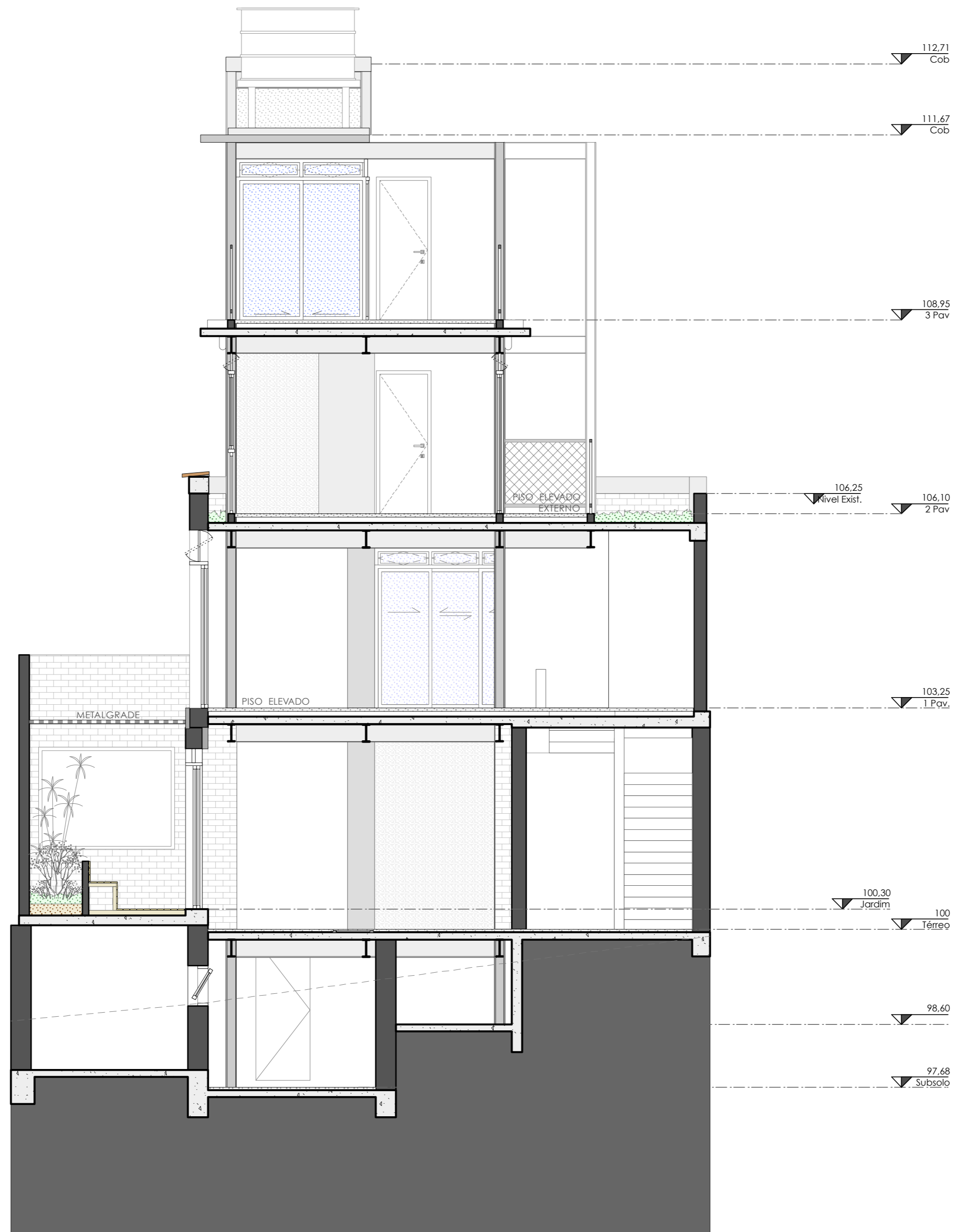
CORTE A
